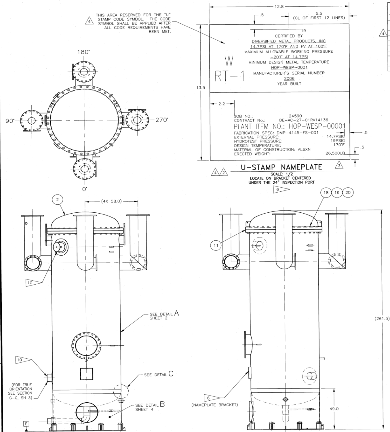
1 VESSEL SUBASSEMBLY SCALE: 1/2" = 1'-0"
