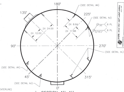
SECTION AH-AH SCALE: 1" = 1'-0"
