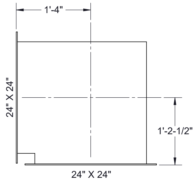
ELBOW W/ TURNING VANES SCALE: 1:12 2 REQD
